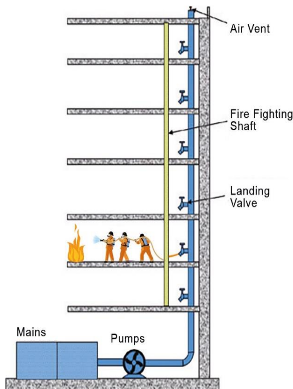
Wet Riser
