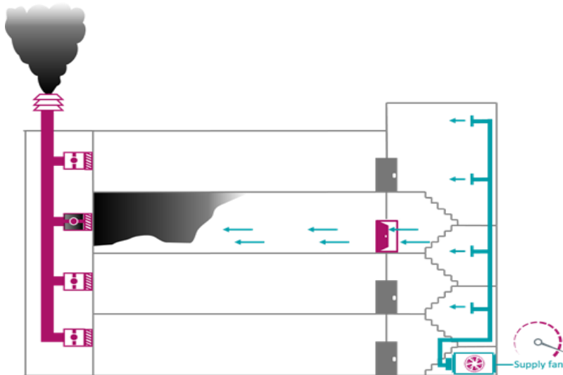
સ્ટેરકેસ પ્રેશ્યુરાઇઝેશન સિસ્ટમ
