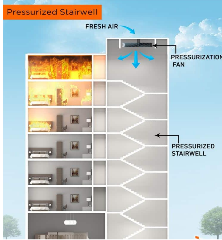
સ્ટેરકેસ પ્રેશ્યુરાઇઝેશન સિસ્ટમ
