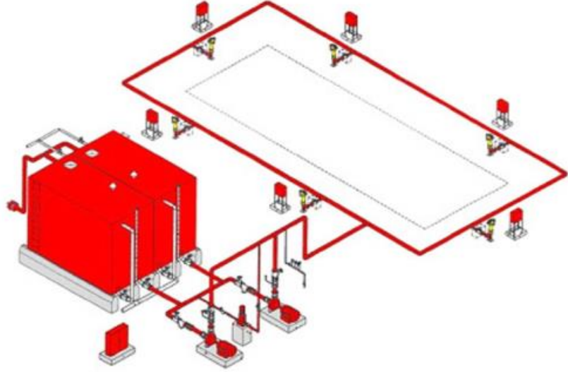
યાર્ડ હાઈડ્રન્ટ
