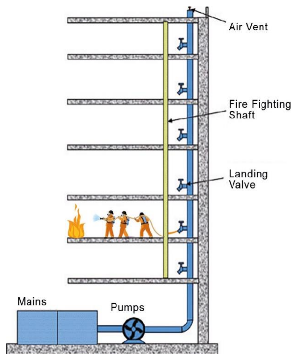
Wet Riser
